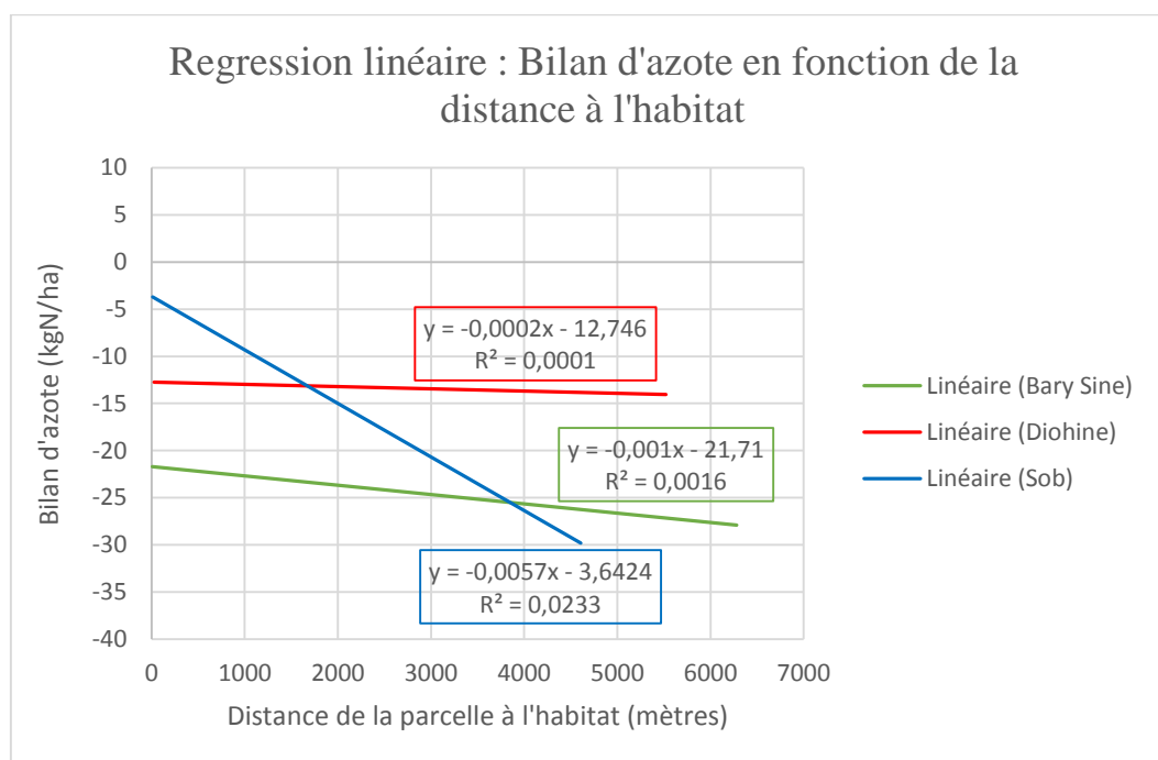
Figure 9 : Régression linéaire des bilans d'azote en fonction de la distance à l'habitat
